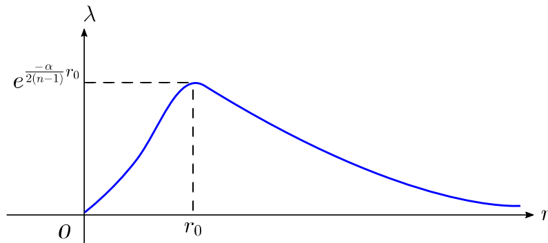
Figura 4 – A função \lambda : [0, +\infty) \rightarrow \mathbb{R} .
