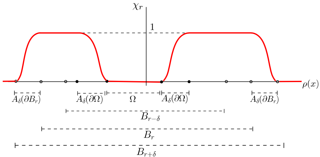
Figura 1 – A função \chi_r com suporte compacto em M \setminus \Omega .
