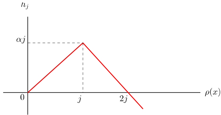
Figura 2 – A função h_j .
