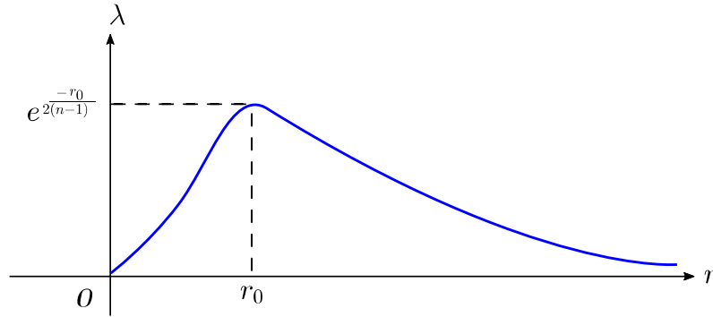
Figura 3 – A função \lambda : [0, +\infty) \rightarrow \mathbb{R} .
